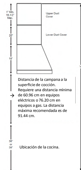
Campanas: ZVW1480SPSS / ZVW1360SPSS / UVW93642PSS
