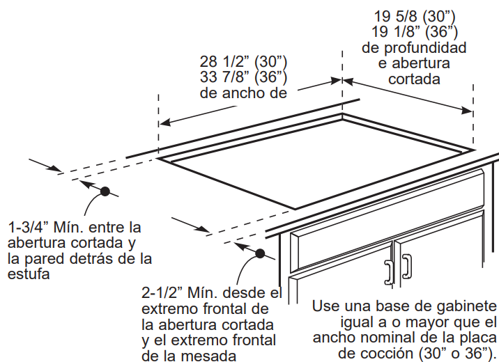
PARRILLA: ZHU36RDTB / ZHU36RTSS
