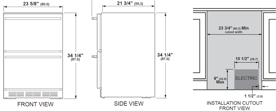
CAJÓN REFRIGERANTE: ZIDI240HII
