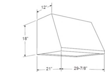
Modelos de 30" Requiere una abertura de 30".
